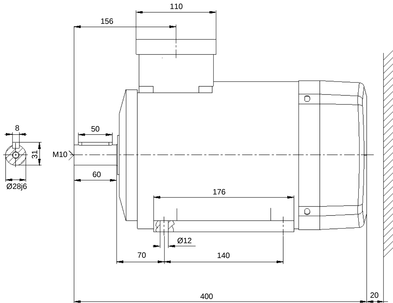
Maßblatt - #306424 - KTE3 112 M 4 KT FL IE3 in Angebot An180204 Position 1 Kabelverschraubung: 2x M25x1,5
